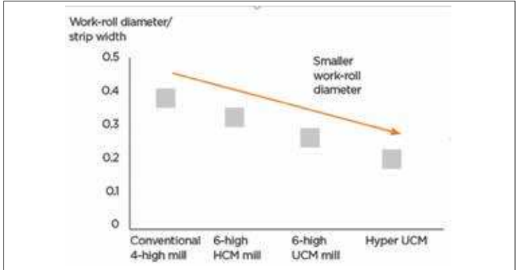
شکل ۲- مقایسه نسبت قطر غلتک نورد به حداکثر عرض ورق در فرایندهای مختلف
