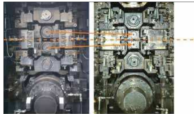
شکل ۲- مقایسه نسبت قطر غلتک نورد در UCM استاندارد و HyperUCM
