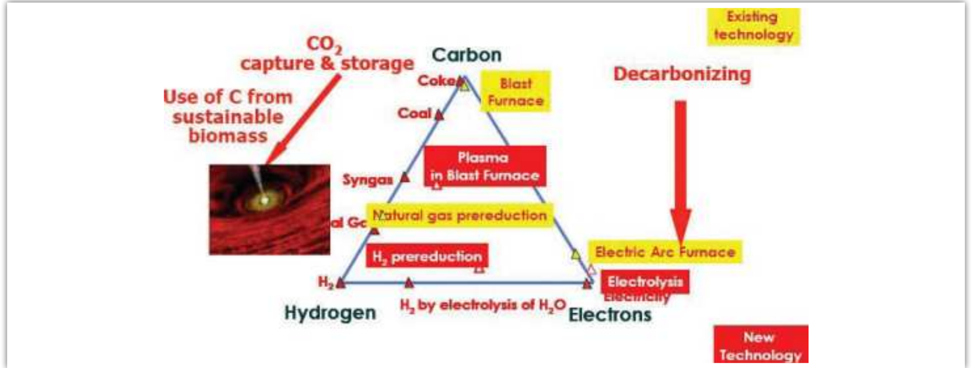
شکل ۲: مسیریهای تکنولوژی‌های پیشرفت برنامه ULCOS.
